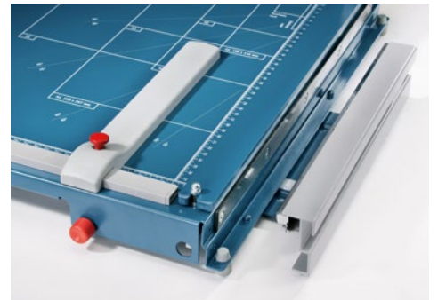
Herausziehbarer Vorderanschlag bis 170 mm mit ausklappbaren Papierhaltern - zum Schneiden von Streifen gleicher Schnittbreite
